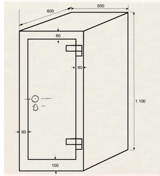
Dibujo acotado Ref. 309 Mod. 1-P
